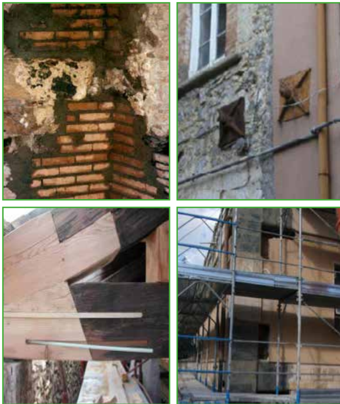
Figura 19. Esempi di intervento (cuci e scuci; capichieve a piastra, rinforzo trave lignea, e fasciature mediante fibre di carbonio) (DPC – ReLUIS, 2011).
